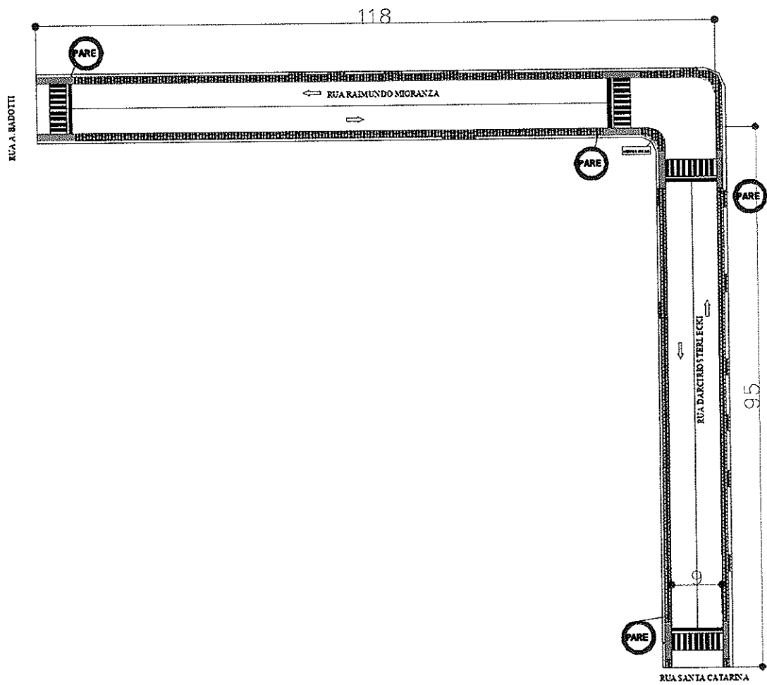
Figura 01 – Cópia de parte do projeto de sinalização de vias.
